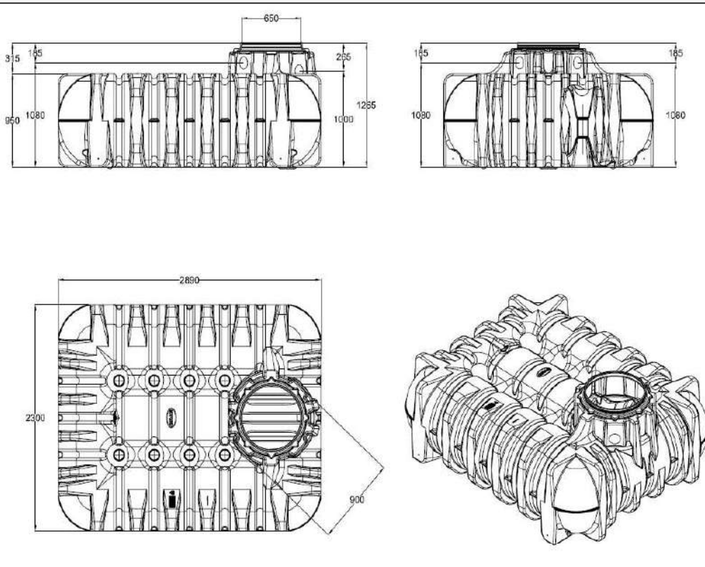
Depósito Platin con cubierta paso peatones
